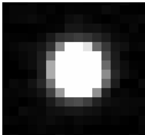
図1. 恒星の拡大
